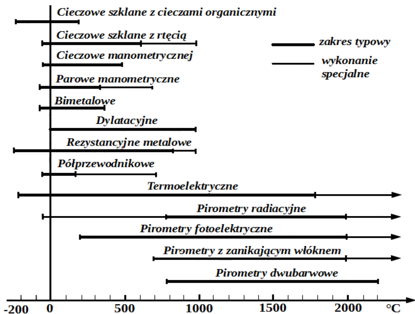
Zakresy stosowania przyrządów do pomiaru temperatury
