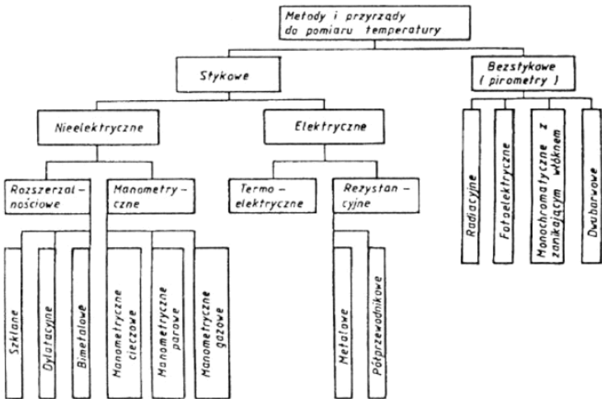
Rys. 1 Klasyfikacja metod i przyrządów do pomiaru temperatury
